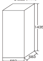
寸法図 (mm)
